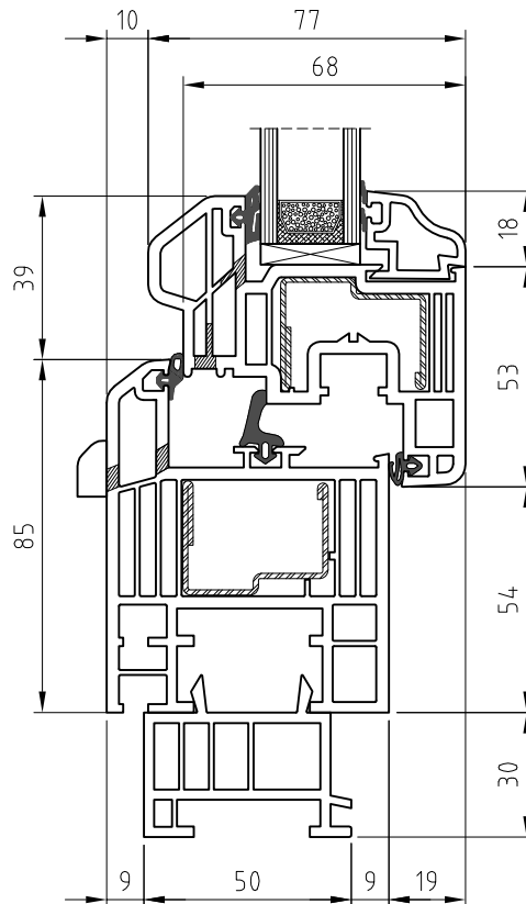
Stock 85 / Flügel 70
