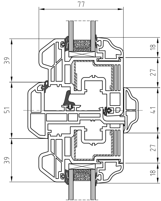
Stulpkämpfer / Flügel 70
