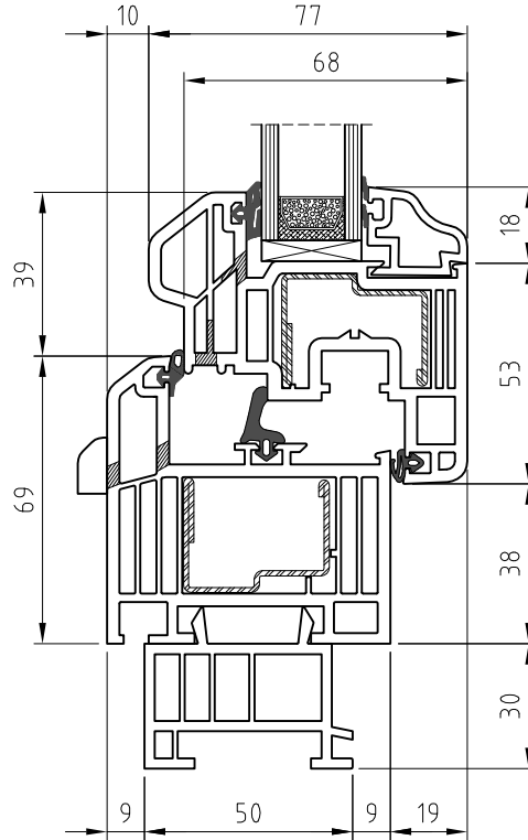
Stock 70 / Flügel 70
