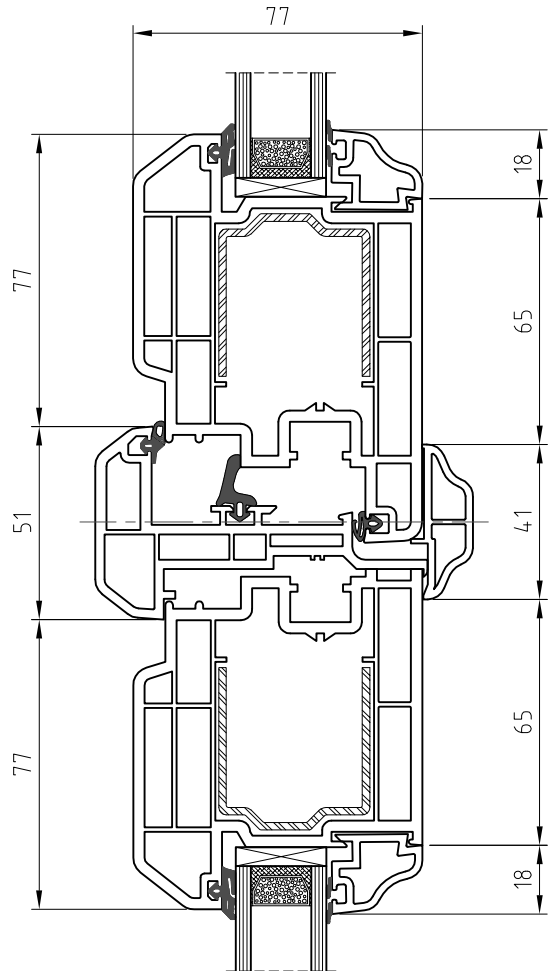
Stulpkämpfer / Flügel 100
